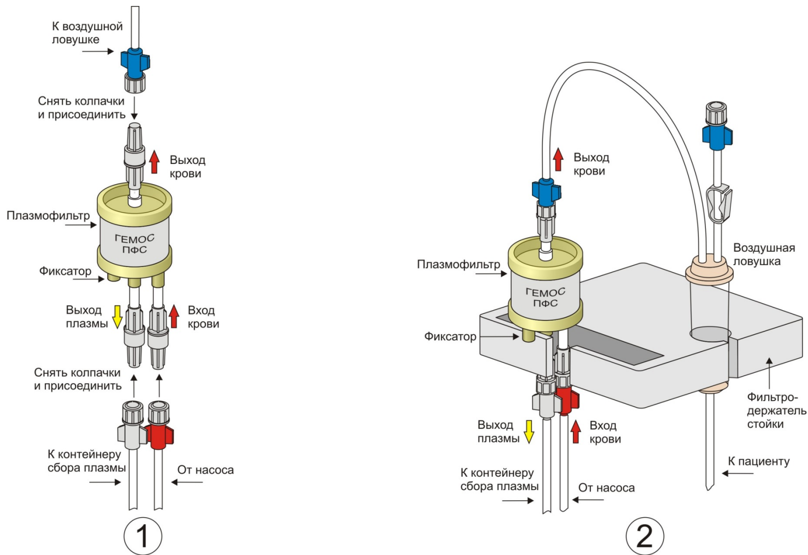
Схема присоединения (1) к магистрали и расположение (2) плазмофильтра «Гемос-ПФС» в фильтродержателе стойки аппарата «Гемофеникс»
